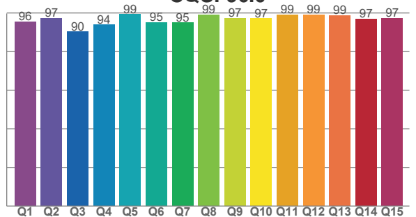
CQS: 96.0
